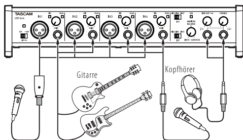
Gesangs-/Sprachmikrofon
